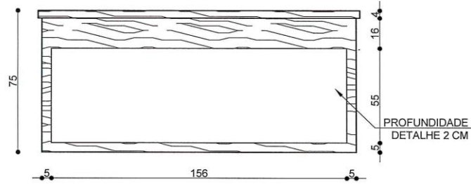
ELEVAÇÃO 02 ESCALA 1/20
