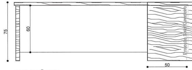
ELEVAÇÃO 03 ESCALA 1/20
