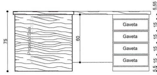
ELEVAÇÃO 04 ESCALA 1/20
