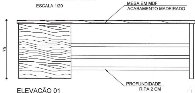
ELEVAÇÃO 01 ESCALA 1/20
